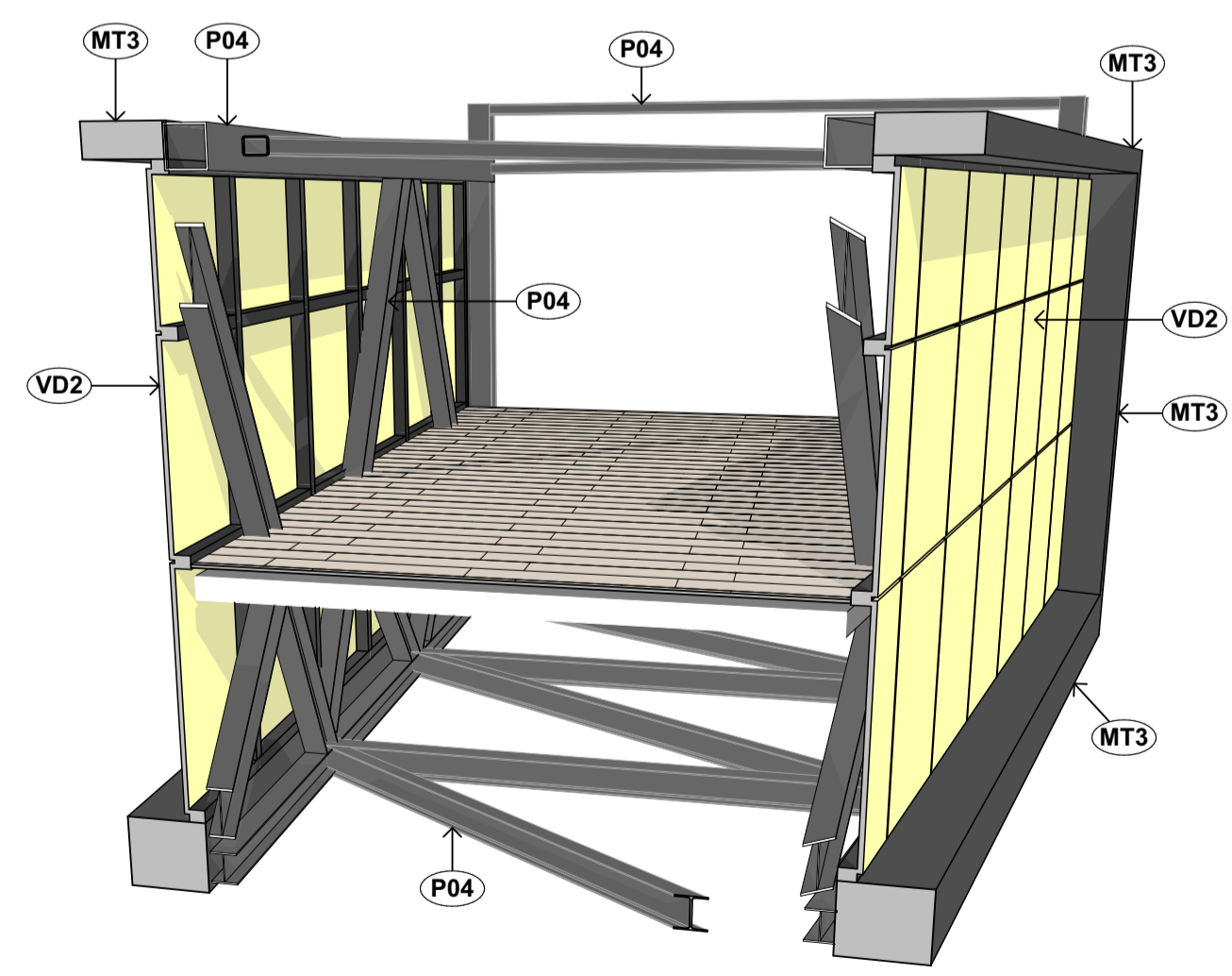
DET. 04
